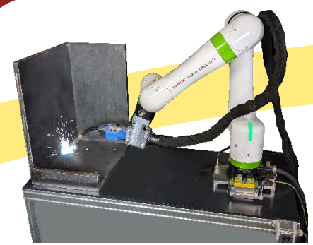
ポータブル協働ロボット CRX-5iA
