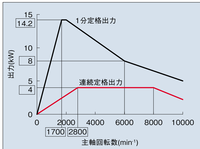
センタースルークーラント仕様
