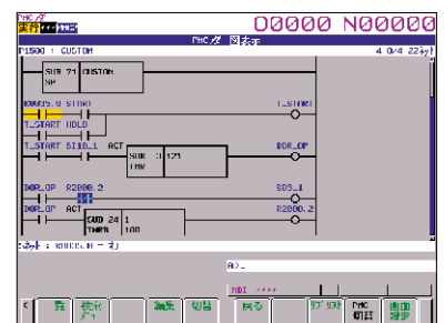
ラダー図表示画面
