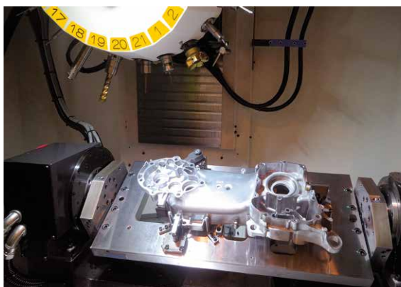
DDR-Ti を使用した割出部品加工の例
